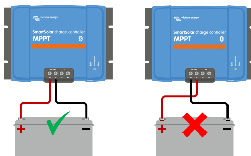
Exemple de inversare corectă și incorectă a polarității bateriei
