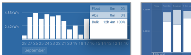
Sistemul rămâne tot timpul în etapa viteză cu defalcare a etapelor de încărcare - Sistem în viteză și absorbție
