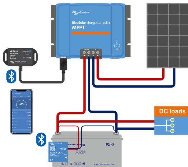
Exemplu de rețea VE.Smart și un Smart Battery Sense și un încărcător solar
